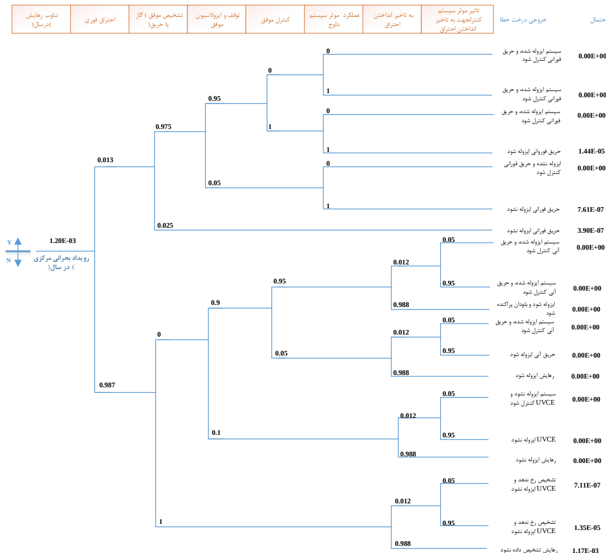
شکل ۱۲ - نمونه درخت رویداد برای سناریوی ره‌ایش در تاسیسات فرایندی
